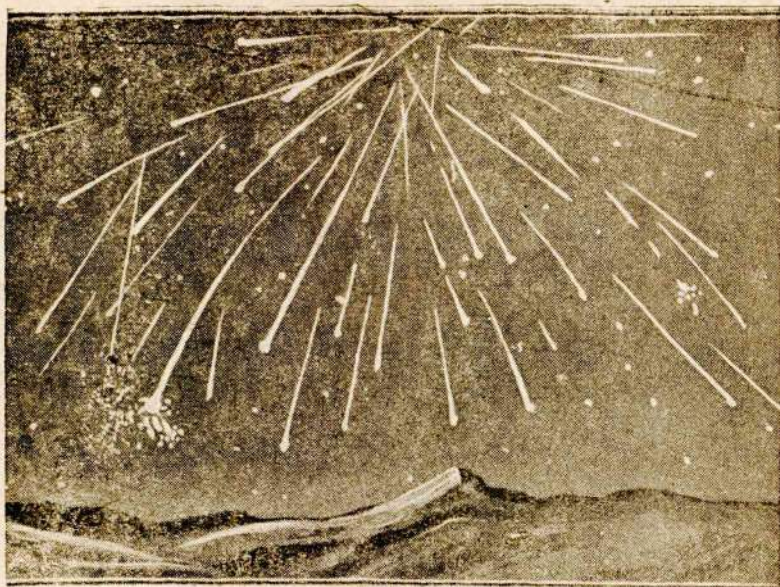
Рис. 11. Дождь падающих звезд, наблюдавшийся в 1872 г. при встрече земли с остатками кометы Биелы
