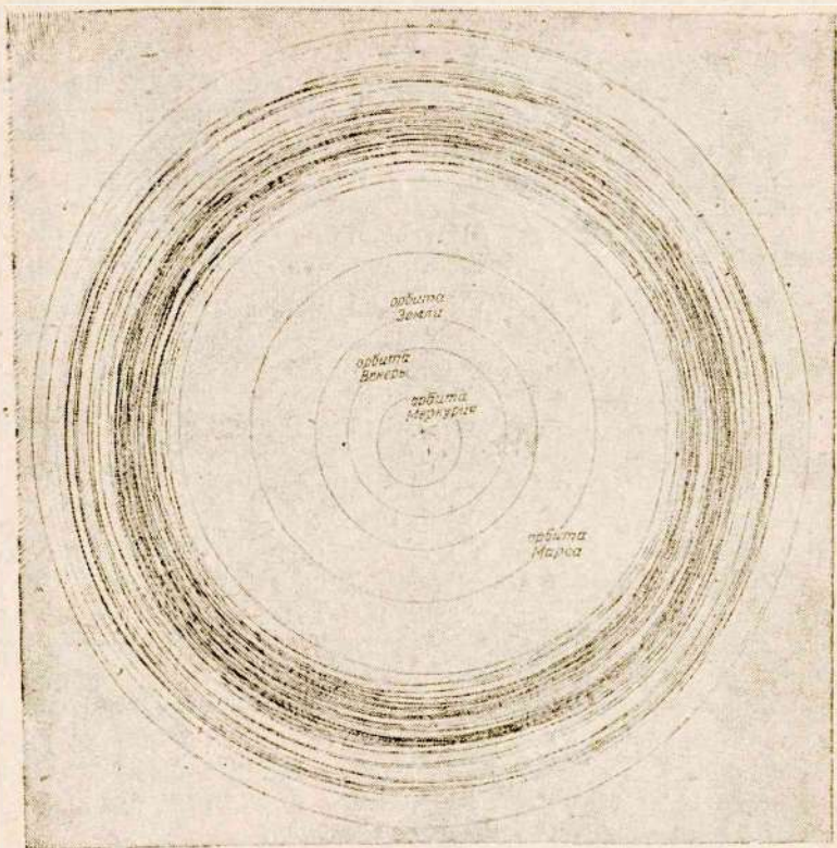
Рис. 3. Орбиты внутренних планет
