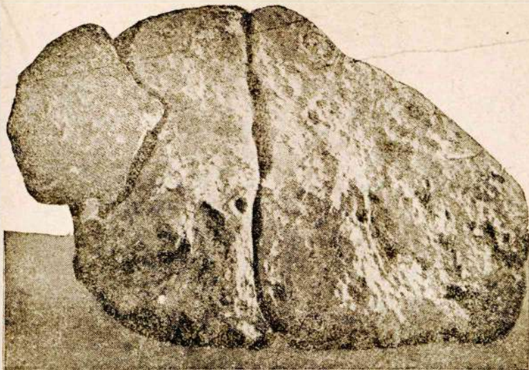
Рис. 9. Метеорит, упавший в Венгрии в 1866 г.
