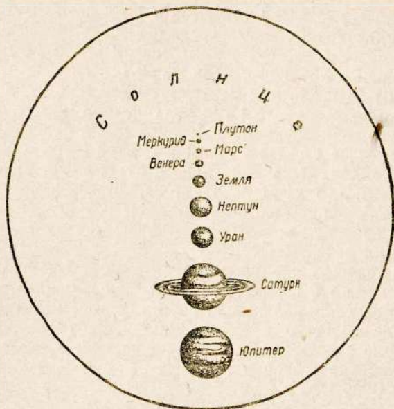
Рис. 1. Сравнительные размеры тел солнечной системы
