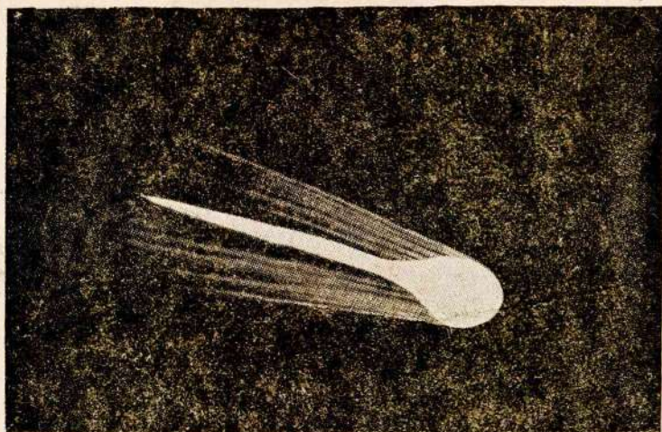
Рис. 8. Болид летящий в земной атмосфере
