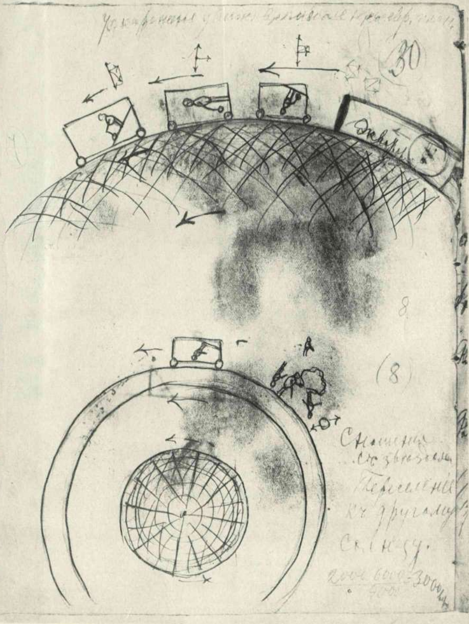
В свободном от тяжести пространстве криволинейное движение производит относительную тяжесть, пропорциональную кривизне дуги и квадрату скорости вагона
