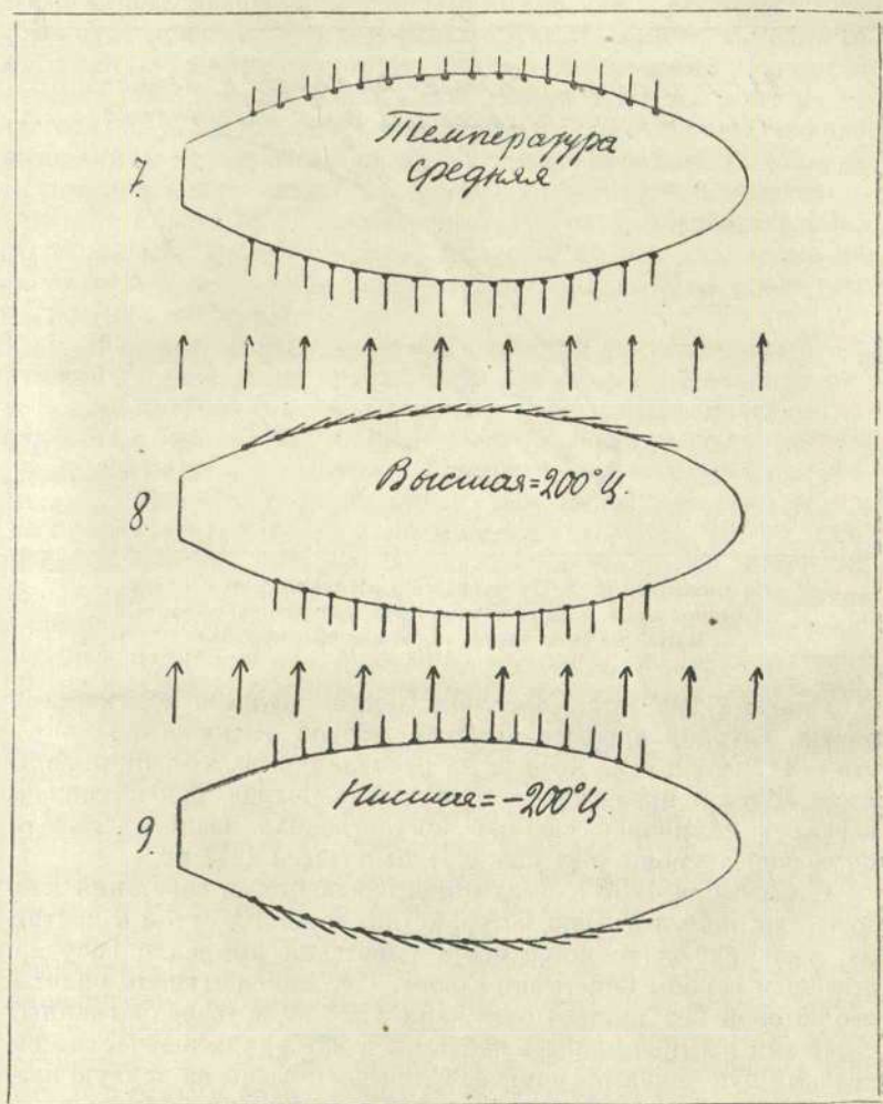
Из рукописи К. Э. Циолковского «Альбом космических путешествий» (1933 г.). Эскиз иллюстрирует действие жалюзи на космическом корабле, которыми регулируется температура внутри него. Стрелками показано направление лучей Солнца.
