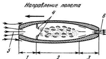
Рис. 5. Схема прямооточного воздушно-реактивного двигателя
