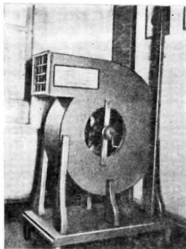
Аэродинамическая груба К. Э. Циолковского («воздуходувка»)
