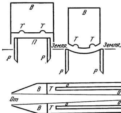
Рис. 11. Чертежи К. Э. Циолковского, поясняющие его идею поезда на воздушной подушке
