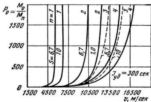
Рис. 19. Зависимость безразмерного полезного груза от скорости для ступенчатых ракет при J_{уд}=300 с.
