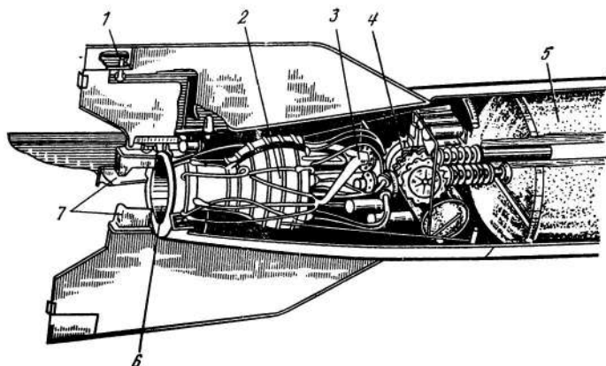
Рис. 4. Жидкостный реактивный двигатель, смонтированный в хвостовой части ракеты
