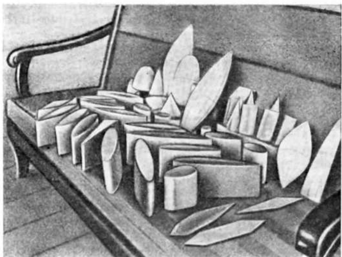
Модели, обследованные К. Э. Циолковским в аэродинамической трубе в г. Калуге в 1897—1901 гг.
