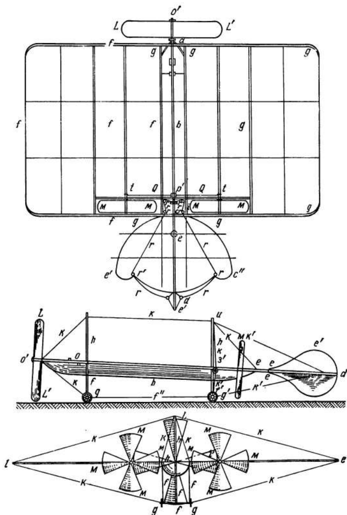
Чертежи аэроплана А. Ф. Можайского
