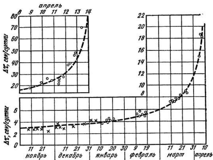
Рис. 23. Изменение периода обращения спутника-2 (СССР) между 3 ноября 1957 г. и 14 апреля 1958 г.
