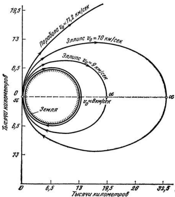
Рис. 22. 0 — точка выхода полезного груза на орбиту; v_0 — скорость, получаемая полезным грузом в точке
