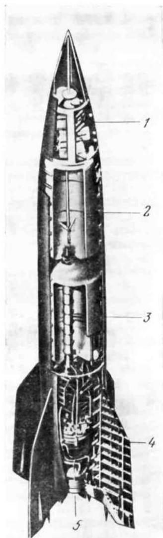
Ракета ФАУ-2
