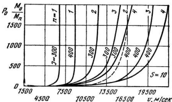
Рис. 20. Зависимость безразмерного полезного груза от скорости для ступенчатых ракет с различной удельной тягой при S=10
