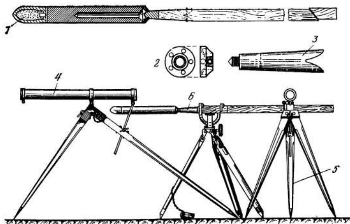
Рис. 6. Детали двухдьюймовой ракеты К. И. Константинова и общий вид ракетного пускового станка
