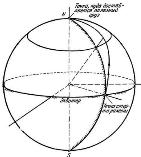
Рис. 13. Оптимальная эллиптическая траектория межконтинентальной ракеты с дальностью полета 10 000 км (влияние атмосферы не учтено)
