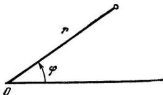
Рис. 21. Полярные координаты ( \gamma, \varphi ) спутника
