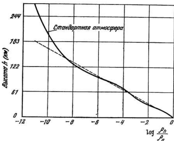
Рис. 27. Сравнение показательного закона изменения плотности воздуха со стандартной атмосферой (по американским данным)
